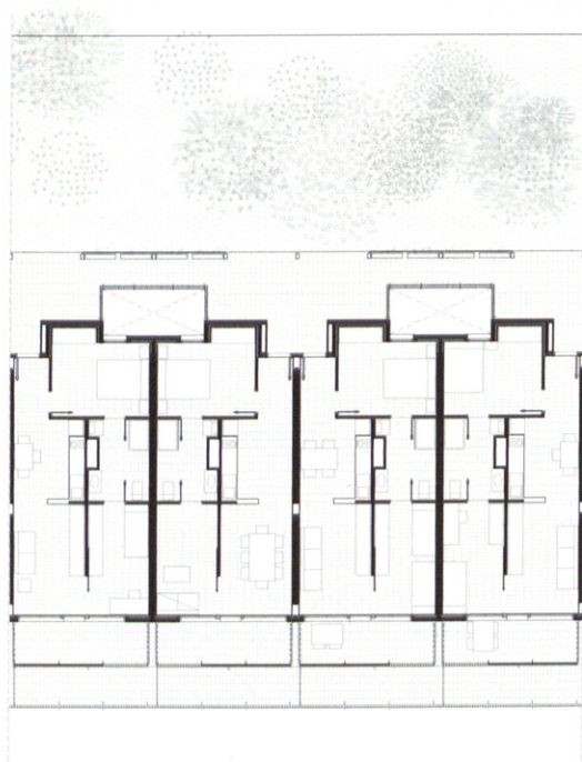
PLANTA TIPO TYPE PLAN
